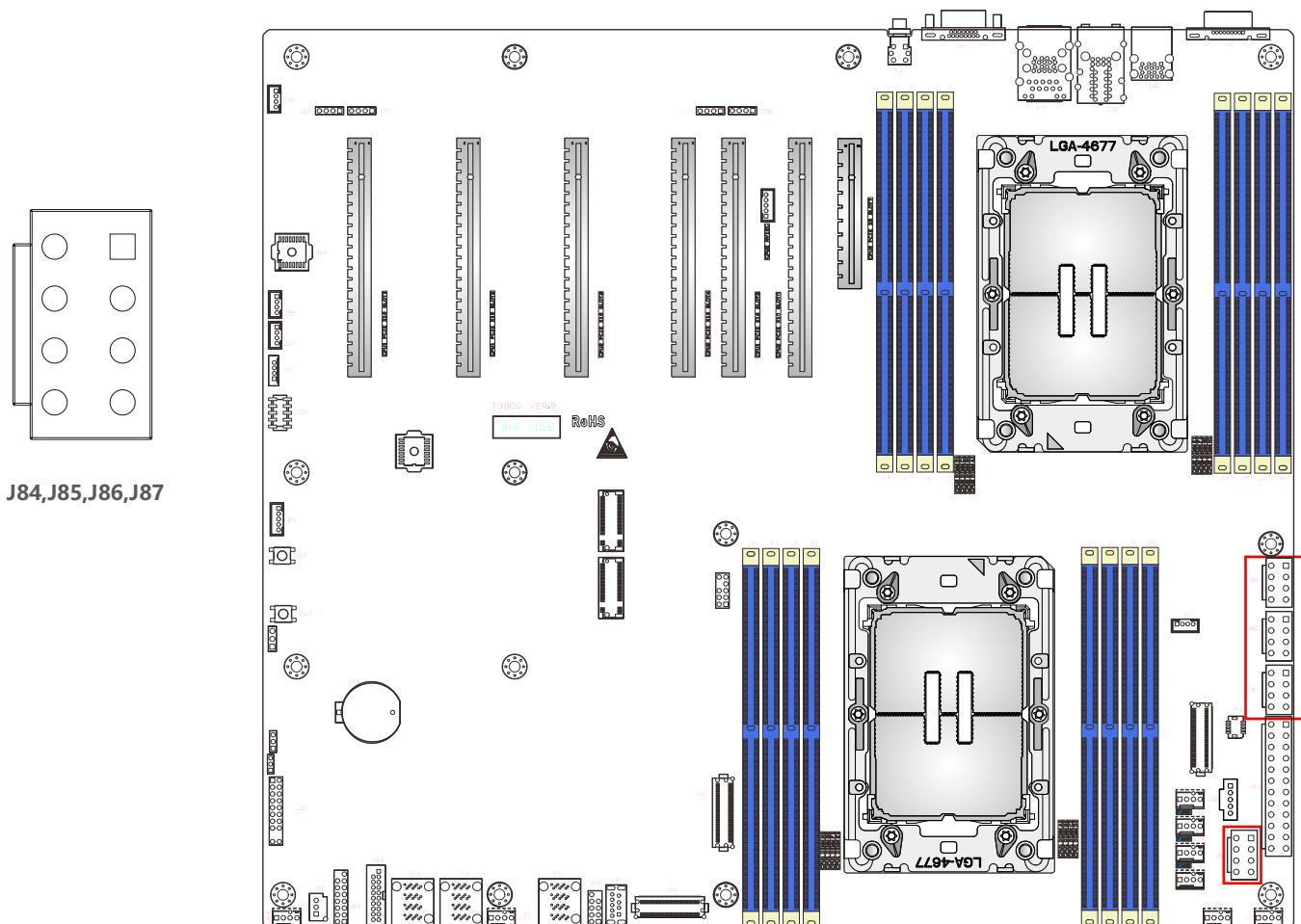
ATX 8Pin (J84, J85, J86, J87)
