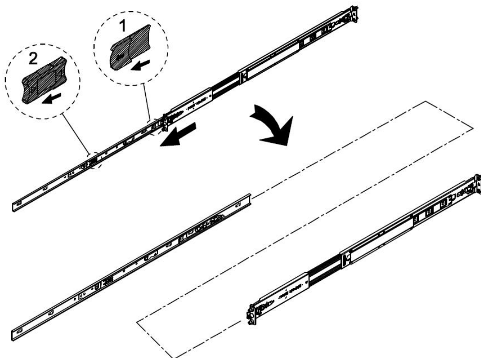
步骤 2. 将内轨安装于主机两侧并锁上螺丝
