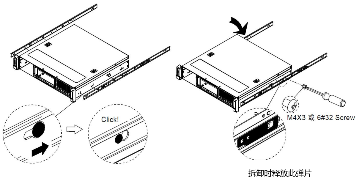
步骤 3. 安装外轨锁上机架
